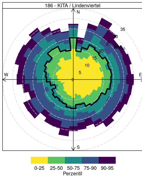
Abb. 20 Verteilung der Schadstoffkonzentrationen nach Windrichtung. Der Median nach Windrichtung wird durch die schwarze Linie angezeigt. Eine starke Ausbuchtung in eine Richtung gibt an, dass es bei Wind aus dieser Richtung gehäuft zu hohen Schadstoffkonzentrationen kommt.
