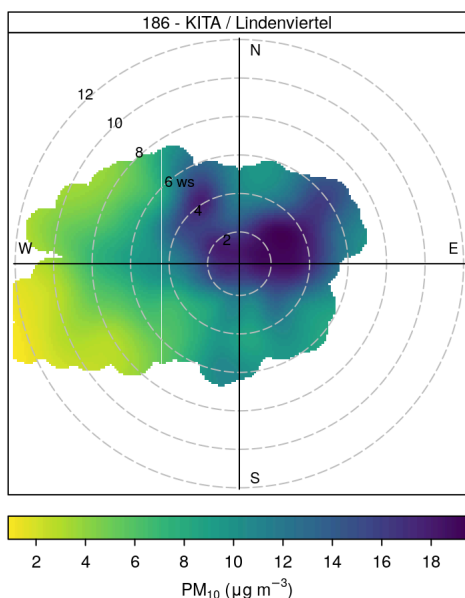
Abb. 21 Mittlere Schadstoffkonzentrationen in Abhängigkeit von Windrichtung und Windgeschwindigkeit. Der Mittelwert der Schadstoffkonzentration wird durch die Farbe angezeigt, die Windstärke durch Entfernung vom Zentrum. Bei lokalen Emissionsquellen sieht man hier meist eine dunkle Färbung im Zentrum, d.h. höhere Schadstoffkonzentrationen bei Windstille. Sieht man eine dunkle Ausbuchtung in eine Richtung deutet dies auf eine entfernte Quelle in dieser Richtung hin, da stärkerer Wind aus dieser Richtung mit höheren Schadstoffkonzentrationen einhergeht.
