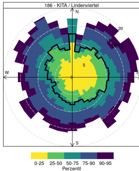
Abb. 15 Verteilung der Schadstoffkonzentrationen nach Windrichtung. Der Median nach Windrichtung wird durch die schwarze Linie angezeigt. Eine starke Ausbuchtung in eine Richtung gibt an, dass es bei Wind aus dieser Richtung gehäuft zu hohen Schadstoffkonzentrationen kommt.
