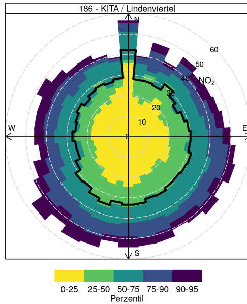
Abb. 5 Verteilung der Schadstoffkonzentrationen nach Windrichtung. Der Median nach Windrichtung wird durch die schwarze Linie angezeigt. Eine starke Ausbuchtung in eine Richtung gibt an, dass es bei Wind aus dieser Richtung gehäuft zu hohen Schadstoffkonzentrationen kommt.
