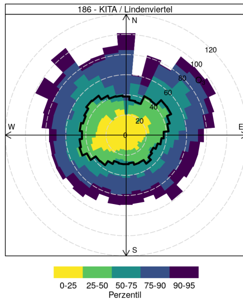
Abb. 10 Verteilung der Schadstoffkonzentrationen nach Windrichtung. Der Median nach Windrichtung wird durch die schwarze Linie angezeigt. Eine starke Ausbuchtung in eine Richtung gibt an, dass es bei Wind aus dieser Richtung gehäuft zu hohen Schadstoffkonzentrationen kommt.
