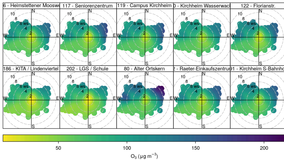
Abb. 11 Mittlere Schadstoffkonzentrationen in Abhängigkeit von Windrichtung und Windgeschwindigkeit.
