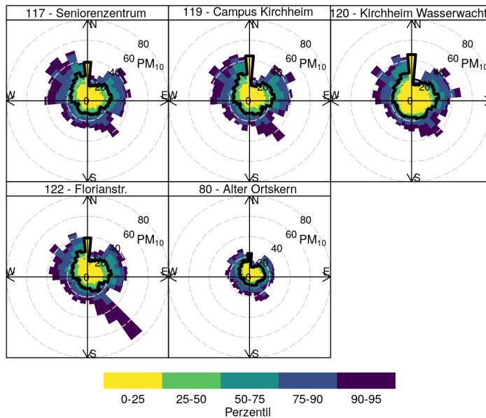
Abb. 20 Verteilung der Schadstoffkonzentrationen nach Windrichtung. Der Median nach Windrichtung wird durch die schwarze Linie angezeigt. Eine starke Ausbuchtung in eine Richtung gibt an, dass es bei Wind aus dieser Richtung gehäuft zu hohen Schadstoffkonzentrationen kommt.
