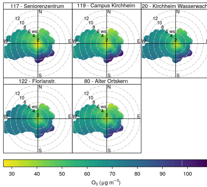
Abb. 11 Mittlere Schadstoffkonzentrationen in Abhängigkeit von Windrichtung und Windgeschwindigkeit.
