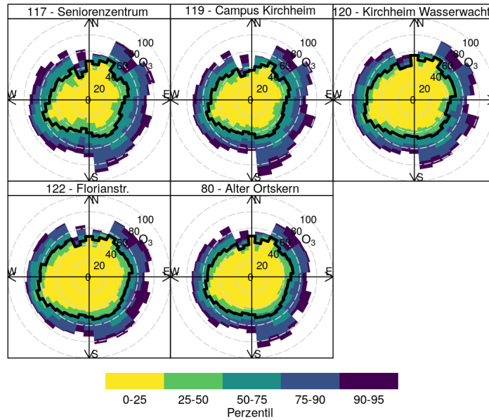
Abb. 10 Verteilung der Schadstoffkonzentrationen nach Windrichtung. Der Median nach Windrichtung wird durch die schwarze Linie angezeigt. Eine starke Ausbuchtung in eine Richtung gibt an, dass es bei Wind aus dieser Richtung gehäuft zu hohen Schadstoffkonzentrationen kommt.
