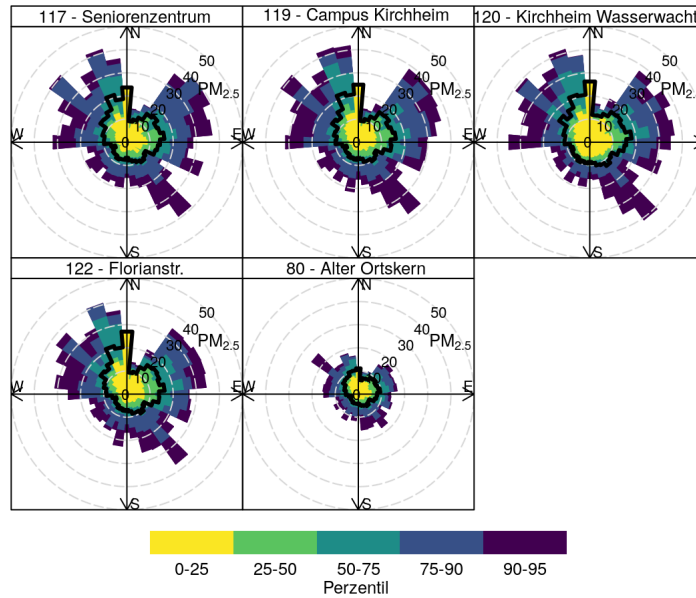
Abb. 15 Verteilung der Schadstoffkonzentrationen nach Windrichtung. Der Median nach Windrichtung wird durch die schwarze Linie angezeigt. Eine starke Ausbuchtung in eine Richtung gibt an, dass es bei Wind aus dieser Richtung gehäuft zu hohen Schadstoffkonzentrationen kommt.
