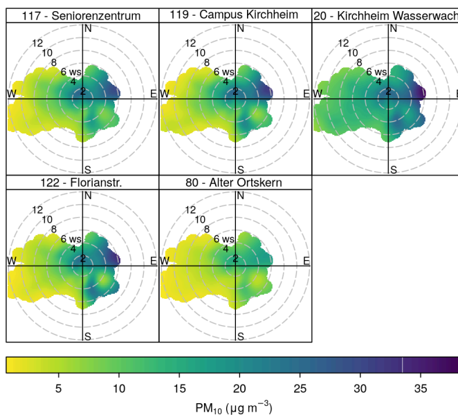
Abb. 21 Mittlere Schadstoffkonzentrationen in Abhängigkeit von Windrichtung und Windgeschwindigkeit. Der Mittelwert der Schadstoffkonzentration wird durch die Farbe angezeigt, die Windstärke durch Entfernung vom Zentrum. Bei lokalen Emissionsquellen sieht man hier meist eine dunkle Färbung im Zentrum, d.h. höhere Schadstoffkonzentrationen bei Windstille. Sieht man eine dunkle Ausbuchtung in eine Richtung deutet dies auf eine entfernte Quelle in dieser Richtung hin, da stärkerer Wind aus dieser Richtung mit höheren Schadstoffkonzentrationen einhergeht.
