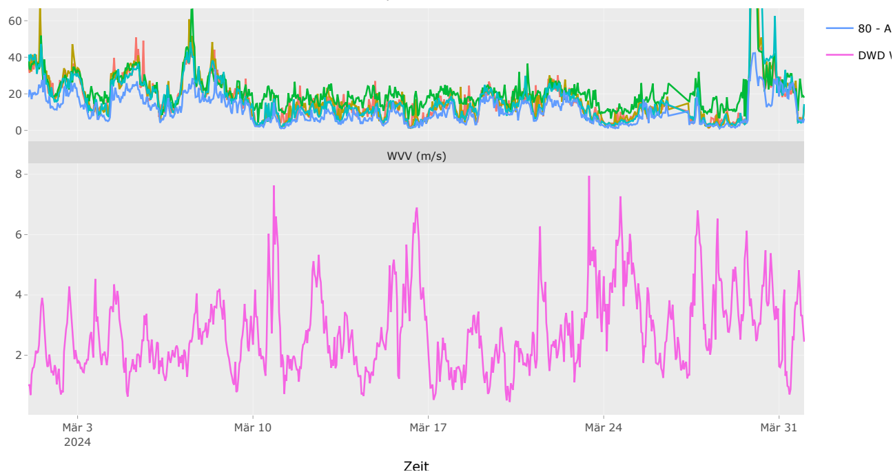
Abb. 18 Zeitlicher Trend der PM_{10} -Konzentrationen mit Wetterparametern. Wetterbedingungen können einen starken Einfluss auf die ambienten Luftschadstoffkonzentrationen haben, z.B. zeigen sich bei starkem Wind meist niedrige Schadstoffkonzentrationen.
