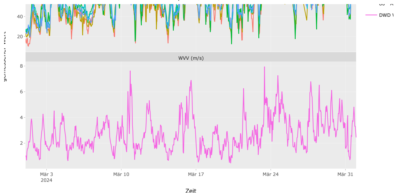
Abb. 8 Zeitlicher Trend der O 3 -Konzentrationen mit Wetterparametern. Wetterbedingungen können einen starken Einfluss auf die ambienten Luftschadstoffkonzentrationen haben, z.B. zeigen sich bei starkem Wind meist niedrige Schadstoffkonzentrationen.
