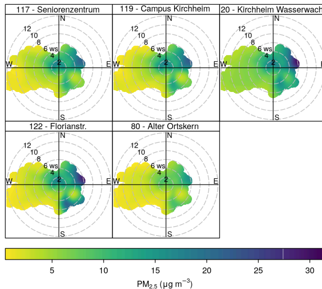
Abb. 16 Mittlere Schadstoffkonzentrationen in Abhängigkeit von Windrichtung und Windgeschwindigkeit. Der Mittelwert der Schadstoffkonzentration wird durch die Farbe angezeigt, die Windstärke durch Entfernung vom Zentrum. Bei lokalen Emissionsquellen sieht man hier meist eine dunkle Färbung im Zentrum, d.h. höhere Schadstoffkonzentrationen bei Windstille. Sieht man eine dunkle Ausbuchtung in eine Richtung deutet dies auf eine entfernte Quelle in dieser Richtung hin, da stärkerer Wind aus dieser Richtung mit höheren Schadstoffkonzentrationen einhergeht.
