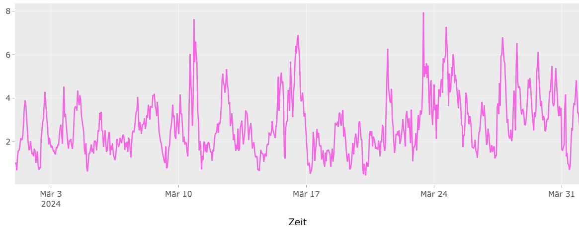
Abb. 13 Zeitlicher Trend der PM_{2.5} -Konzentrationen mit Wetterparametern. Wetterbedingungen können einen starken Einfluss auf die ambienten Luftschadstoffkonzentrationen haben, z.B. zeigen sich bei starkem Wind meist niedrige Schadstoffkonzentrationen.
