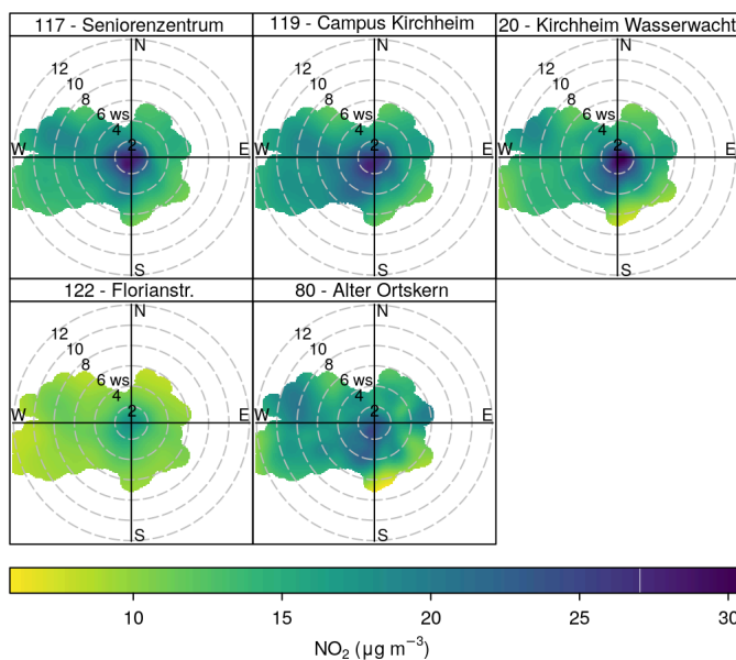
Abb. 6 Mittlere Schadstoffkonzentrationen in Abhängigkeit von Windrichtung und Windgeschwindigkeit. Der Mittelwert der Schadstoffkonzentration wird durch die Farbe angezeigt, die Windstärke durch Entfernung vom Zentrum. Bei lokalen Emissionsquellen sieht man hier meist eine dunkle Färbung im Zentrum, d.h. höhere Schadstoffkonzentrationen bei Windstille. Sieht man eine dunkle Ausbuchtung in eine Richtung deutet dies auf eine entfernte Quelle in dieser Richtung hin, da stärkerer Wind aus dieser Richtung mit höheren Schadstoffkonzentrationen einhergeht.
