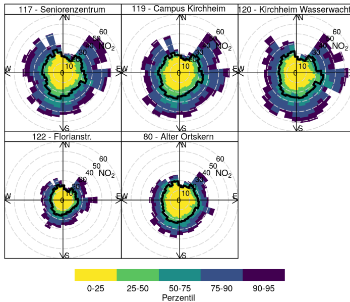
Abb. 5 Verteilung der Schadstoffkonzentrationen nach Windrichtung. Der Median nach Windrichtung wird durch die schwarze Linie angezeigt. Eine starke Ausbuchtung in eine Richtung gibt an, dass es bei Wind aus dieser Richtung gehäuft zu hohen Schadstoffkonzentrationen kommt.
